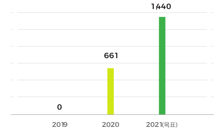
진천 CDC 태양광 에너지 생산량 연간 발전량(Mwh)
